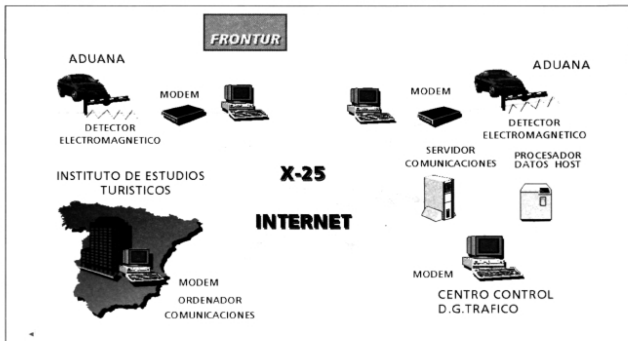
FIGURA 4 Sistema conteo vehículos
